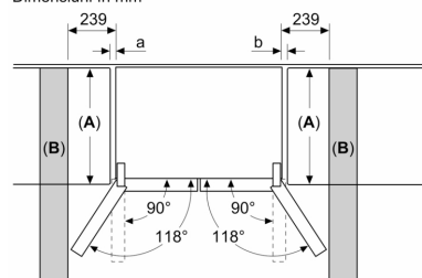
Dimensiuni în mm
