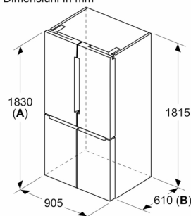
Dimensiuni în mm
