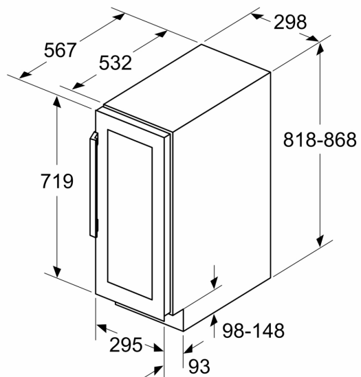
Dimensiuni în mm
